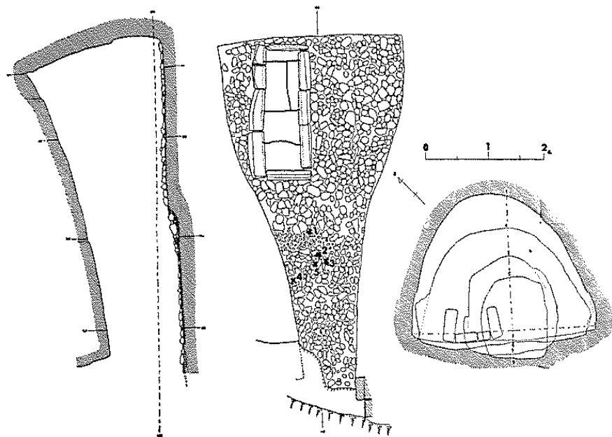
2号墓 全長:5.45m
